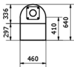
B-B ( 1 : 25 )
